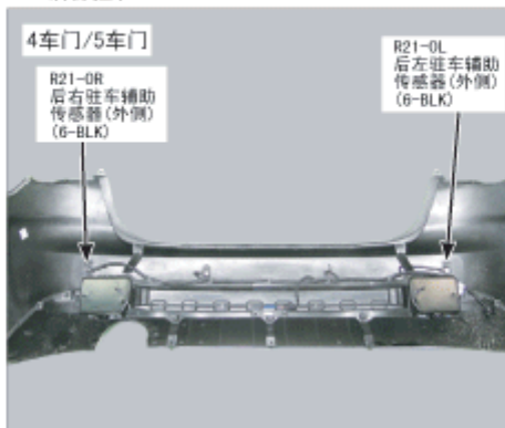
104. 后保险杠
