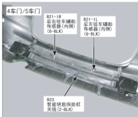
103. 后保险杠
