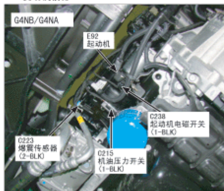
108. 发动机前部
