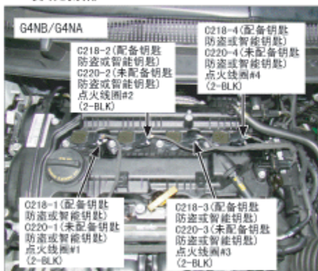
107. 发动机顶部
